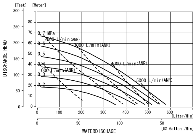
■ NDP-50BPT/BVT
