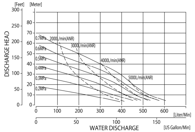
■ NDP-50BAT/BST/BFT
