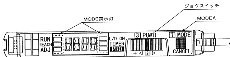
Fig.4.13 アンプ各部の名称
