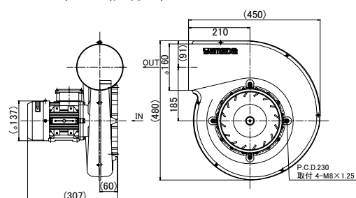
N16 ファン(直付型)
