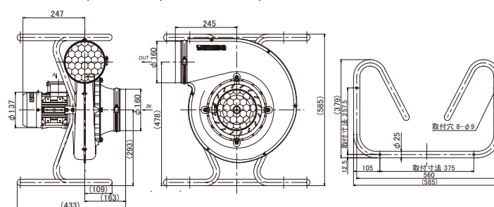
N24 ファン F (フリスカス型)
