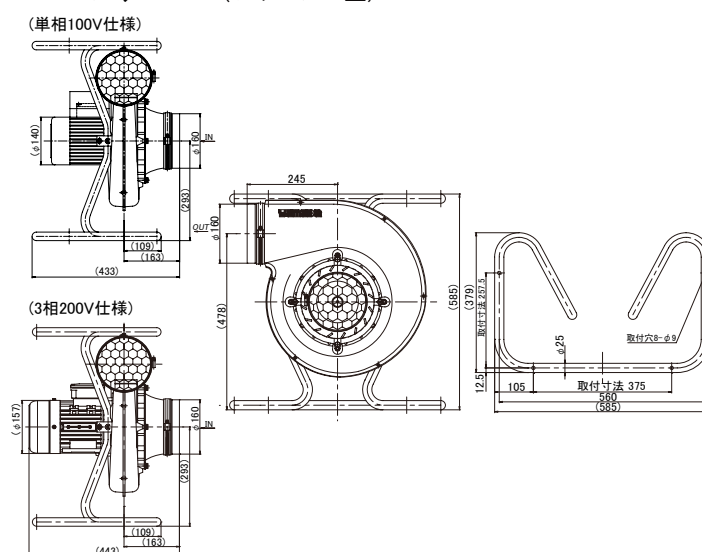
N24 ファン F (フリスカス型)
