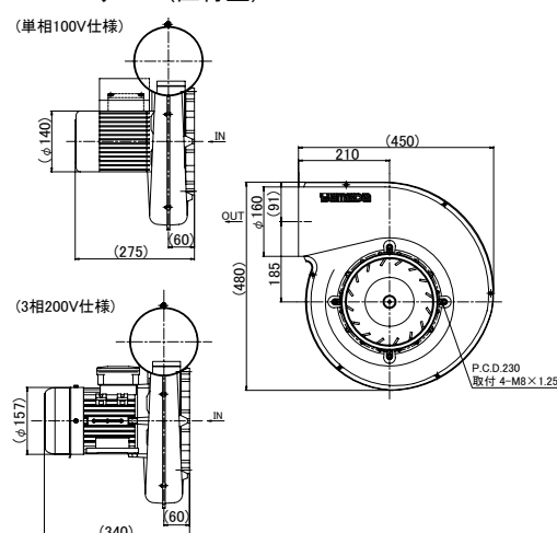
N24 ファン(直付型)
