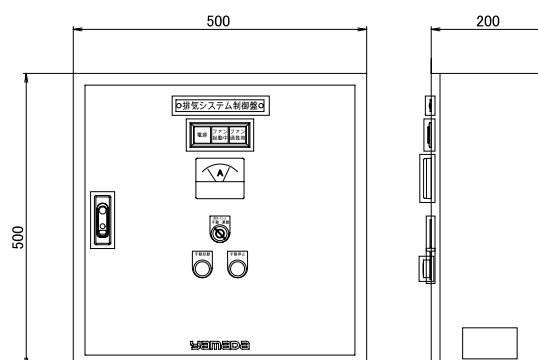
■寸法図
