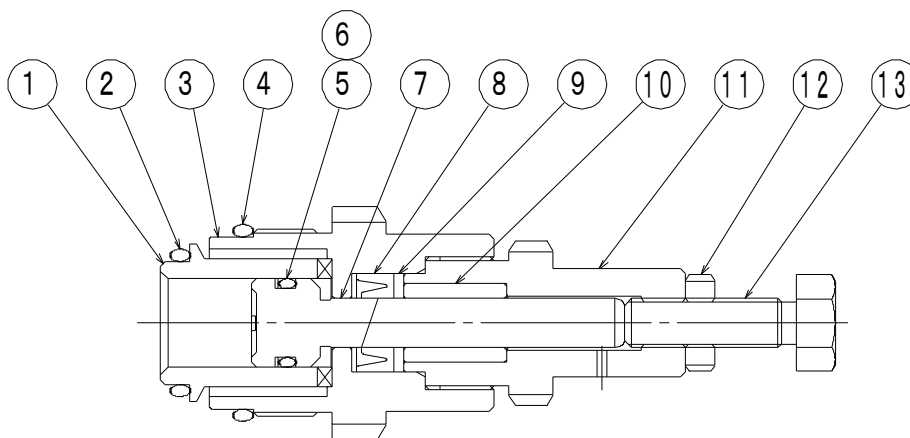
800K858 5mL 定量シリンダ
