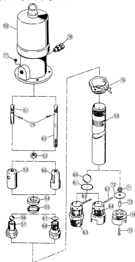
部品分解図 110 型 5 : 1 ポンプシリーズ
