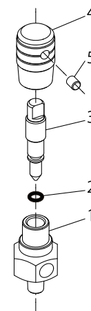
800327 スロットルバルブ 組立
