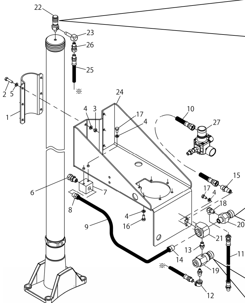
802556 ブラケット組立
