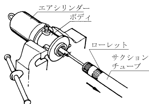
エアモーター Fig.6
