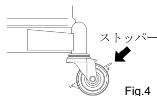
ブレーキ付きキャスター
