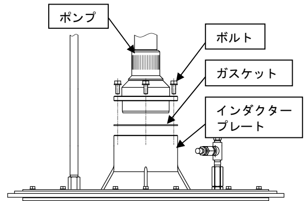
Fig.5 インダクタープレートの取り付け
