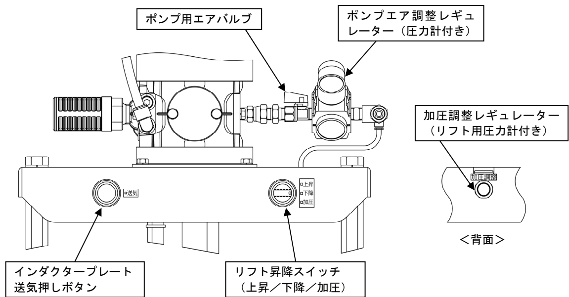
Fig.2 操作部の名称
