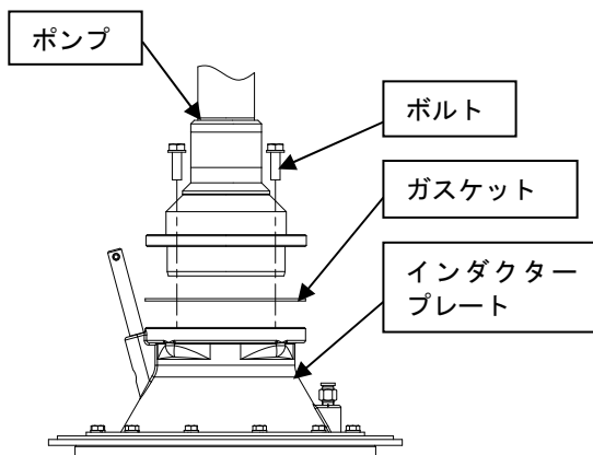
Fig.6 インダクタープレートの取り付け
