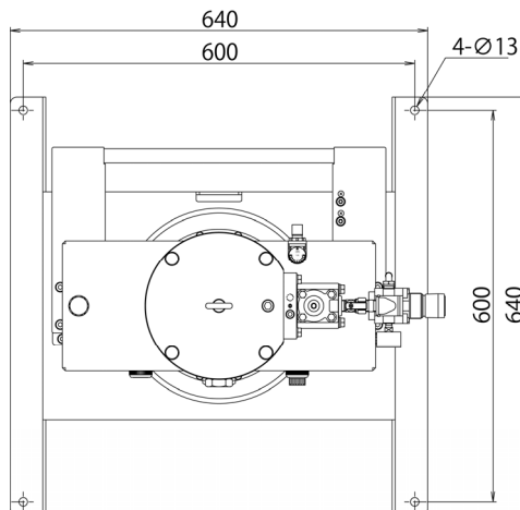
Fig.3 固定使用時の設置寸法
