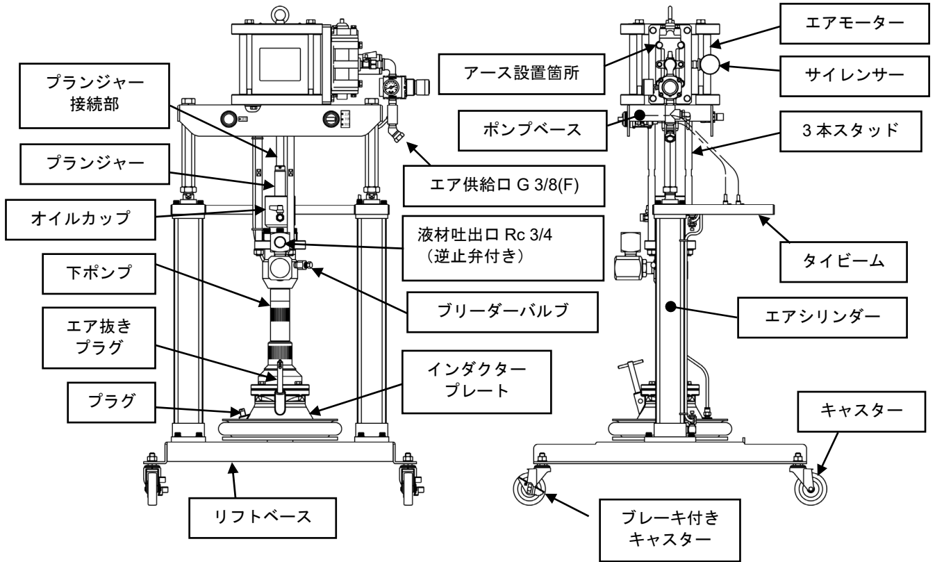
Fig.1 各部の名称
