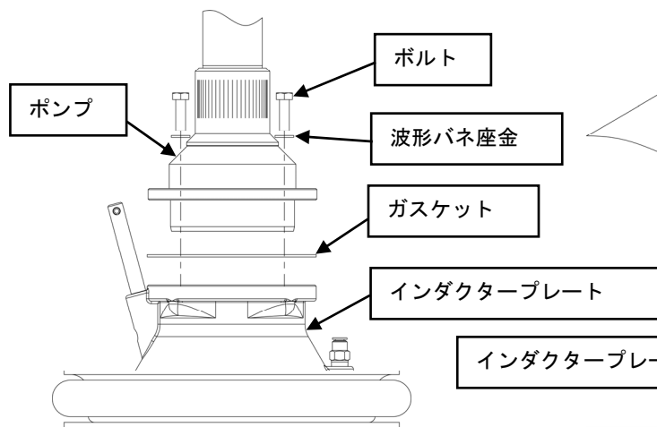
Fig.7 インダクタープレートの取り付け
