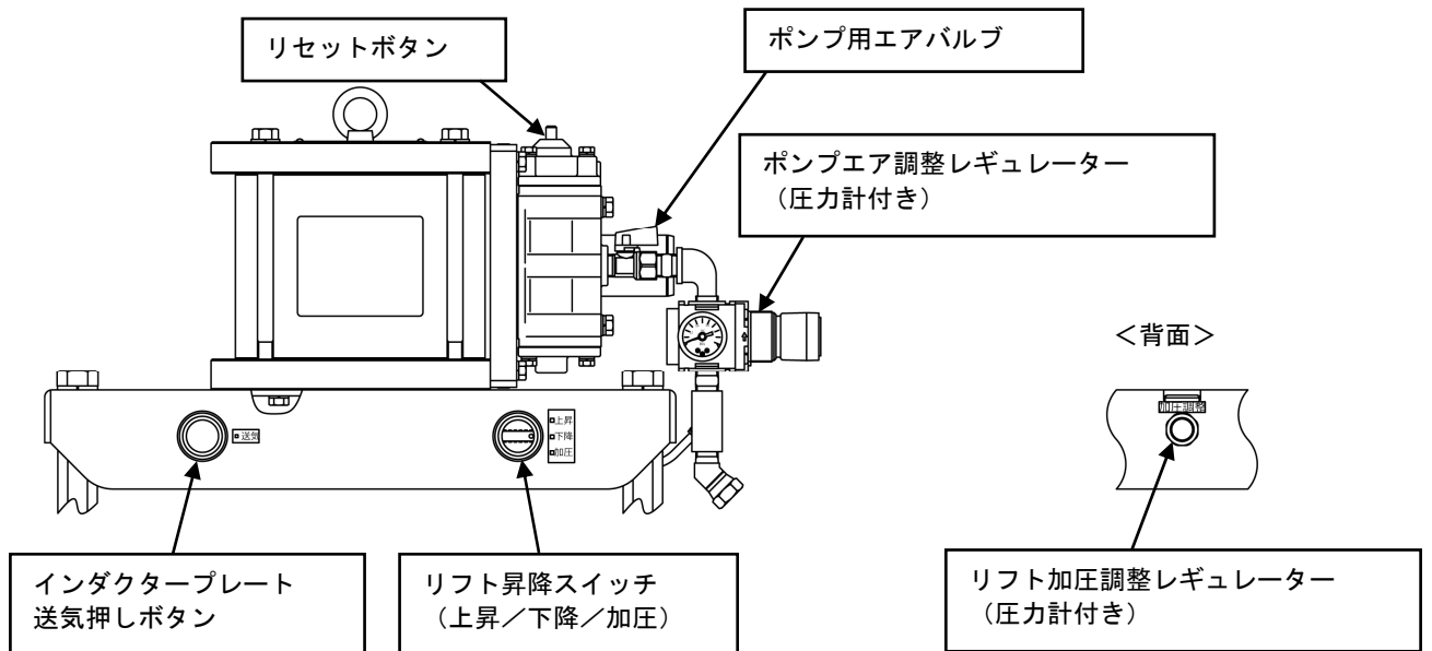
Fig.2 操作部の名称
