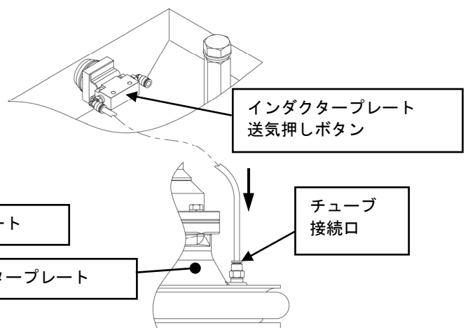
Fig.8 送気用チューブの接続
