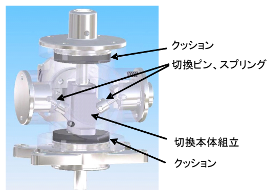
図 2. 切換バルブ内部構造図
