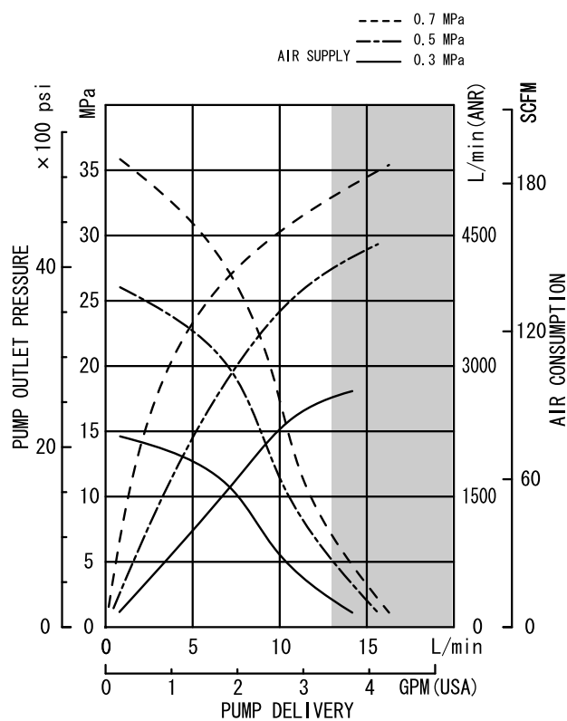
SR250P55 パフォーマンスカーブ
