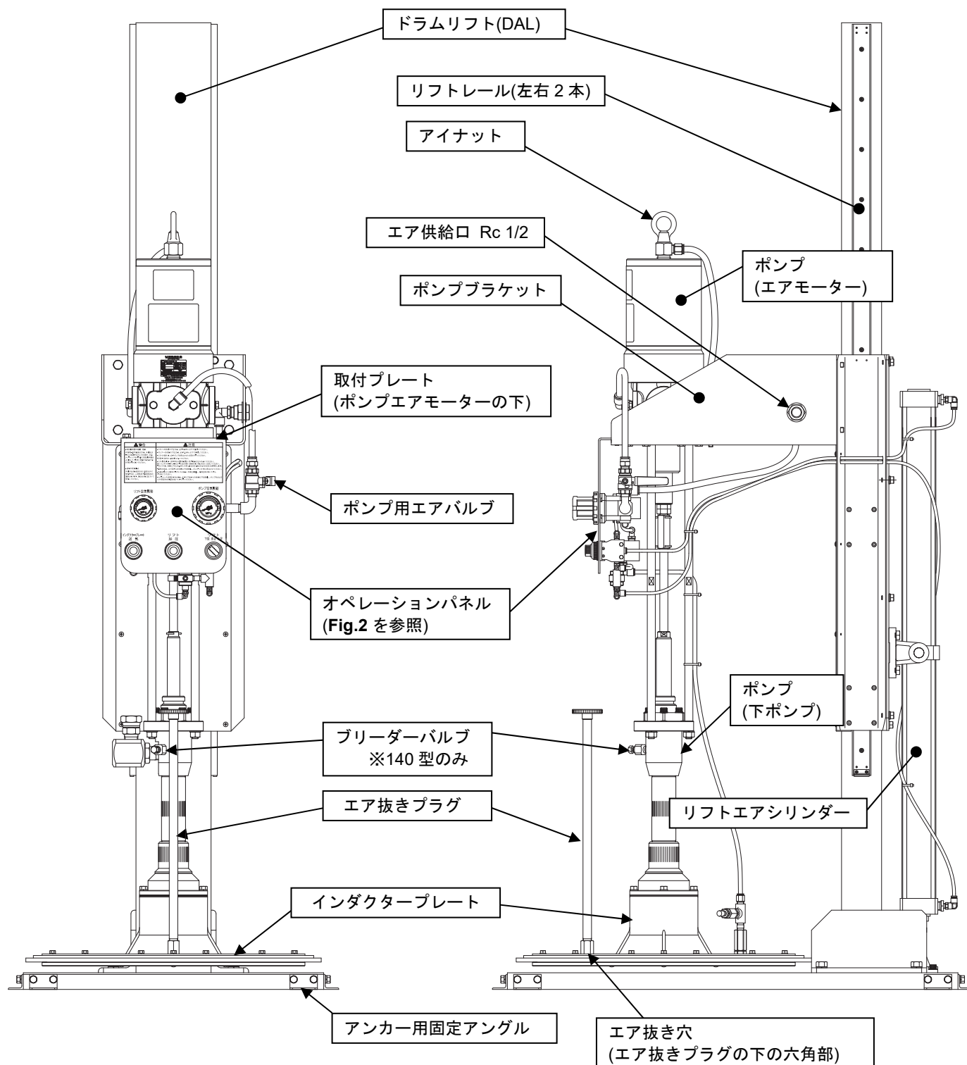
Fig.1 各部の名称
