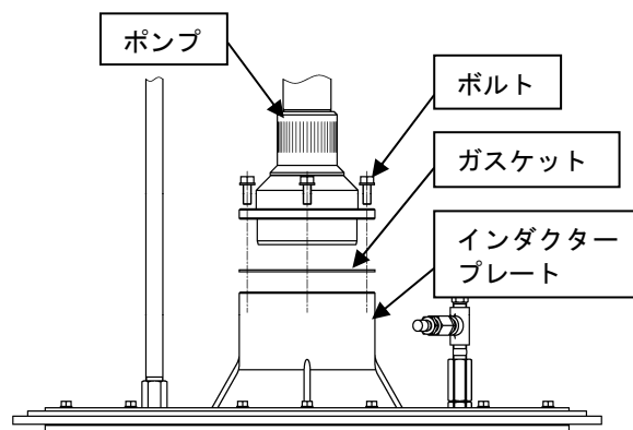
Fig.5 インダクタープレートの取り付け
