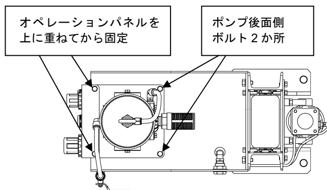
Fig.7 左記 Fig.6 の A 矢視図
