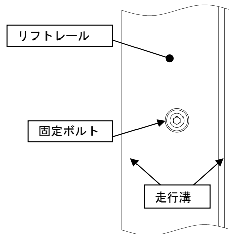
Fig.10 リフトレールの給脂場所
