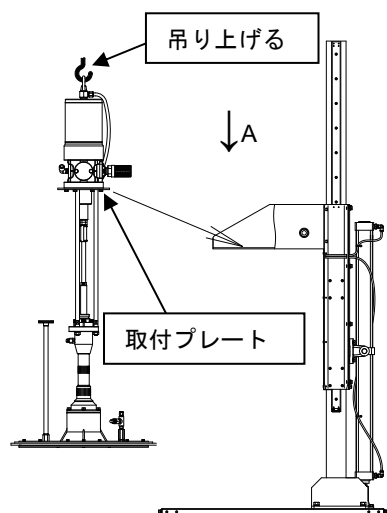
Fig.6 リフトへのポンプ取り付け
