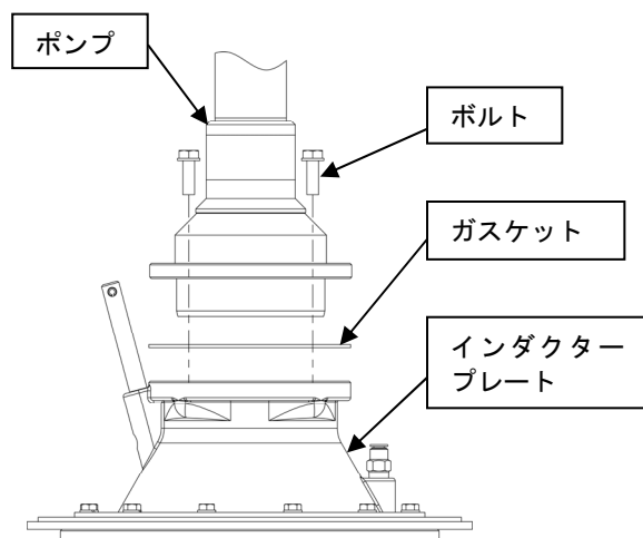
Fig.6 インダクタープレートの取り付け
