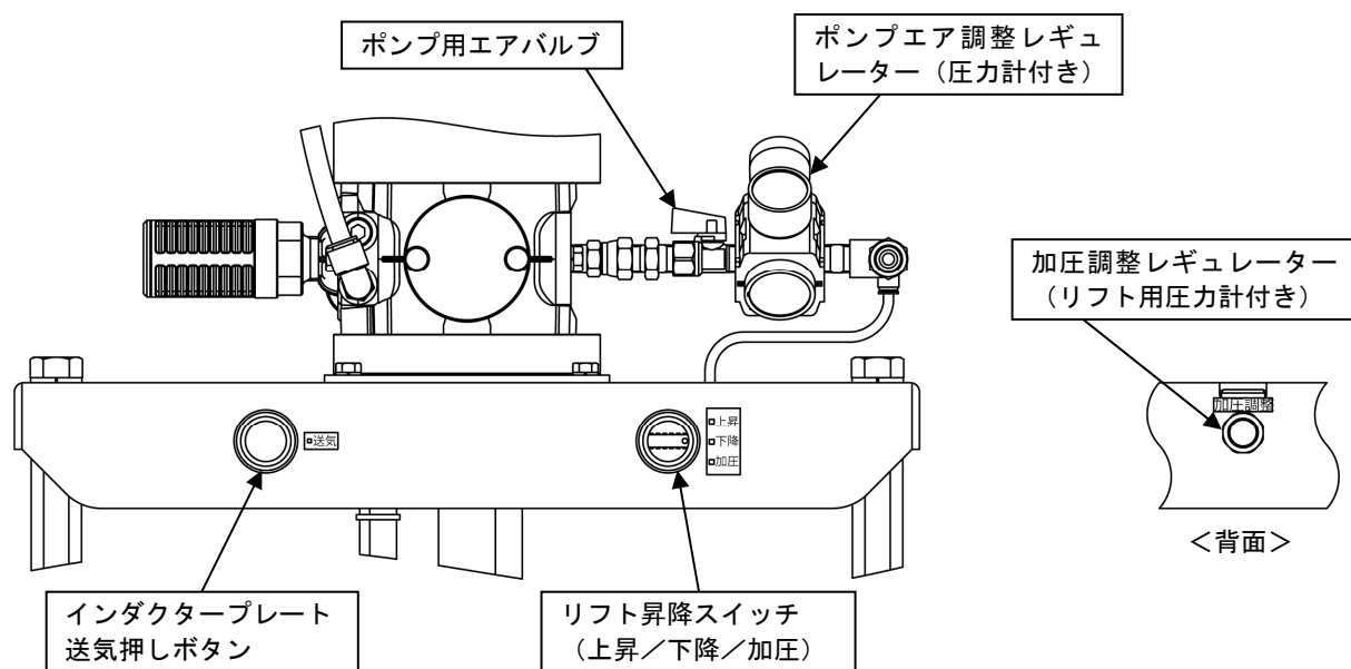
Fig.2 操作部の名称
