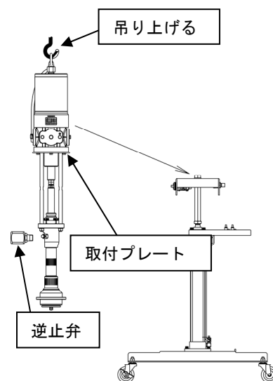
Fig.5 リフトへのポンプ取り付け
