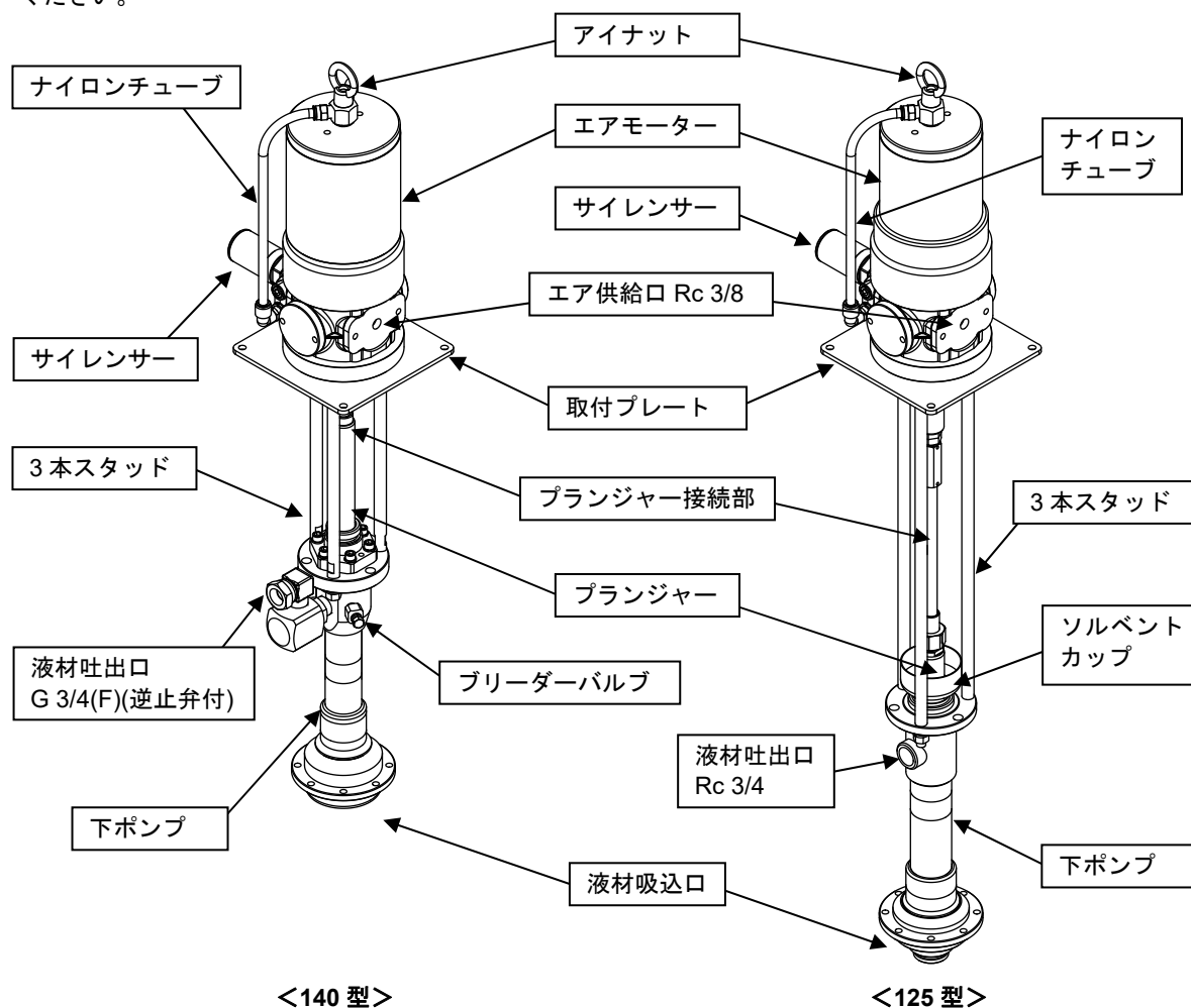
Fig.1 各部の名称
