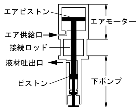
Fig.2 作動原理図
