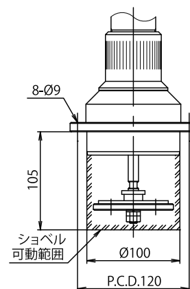
Fig.7 シヨベル可動範囲と取り付け寸法
