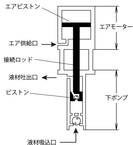
Fig.2 作動原理図
