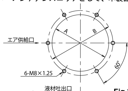
Fig.3 取付寸法
