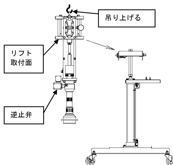
Fig.6 リフトへのポンプ取付
