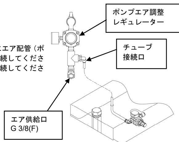
Fig.9 リフト用エア供給チューブの接続
