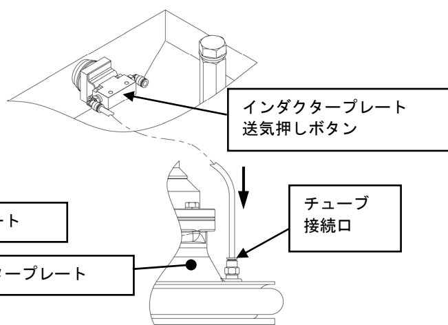
Fig.8 送気用チューブの接続
