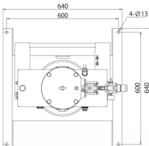
Fig.3 固定使用時の設置寸法
