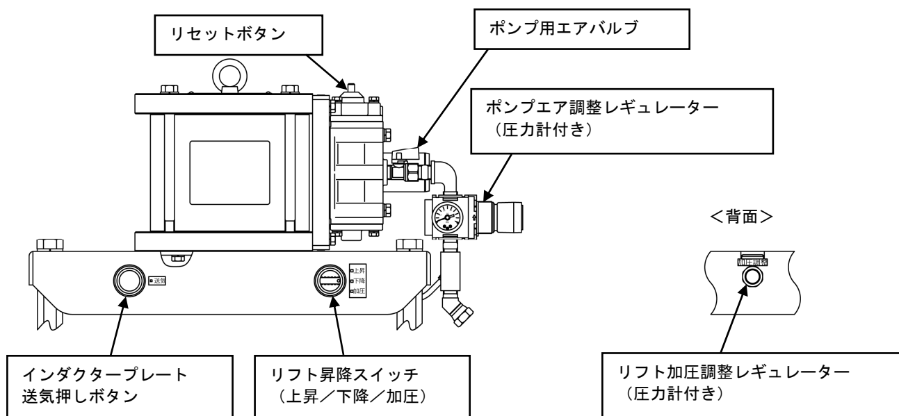
Fig.2 操作部の名称
