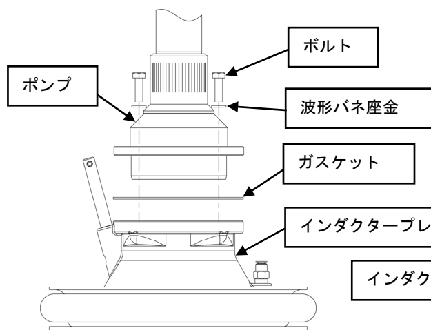
Fig.7 インダクタープレートの取り付け
