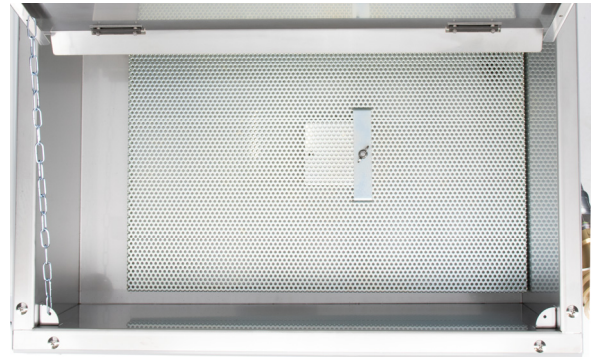
パンチングアミ右寄せ (出荷状態)
