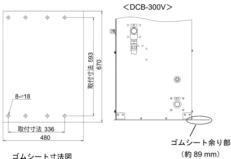
ゴムシート寸法図
