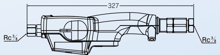
805160 フレキノズルクミタテ NDN-FS-3 (スイベル付)
