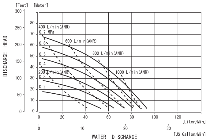
■ NDP-20BA□-D
