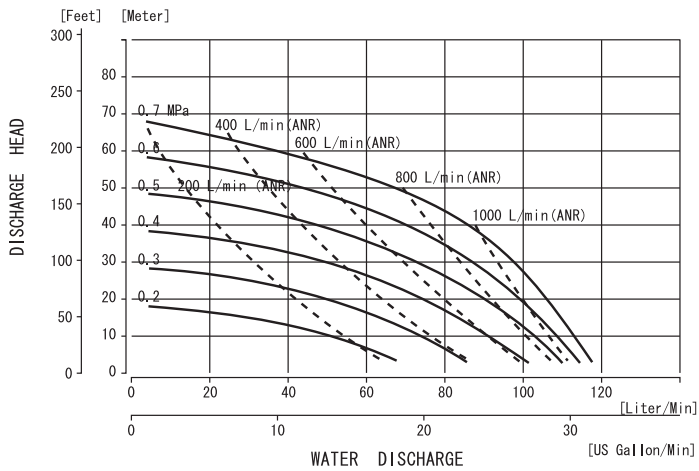
■ NDP-20BA□-D
