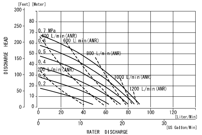
■ NDP-20BAT-D
