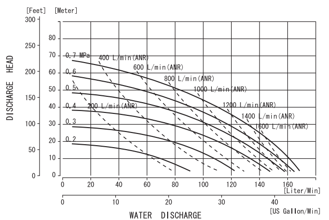
■ NDP-25BAT/BST/BFT/BPT/BVT
