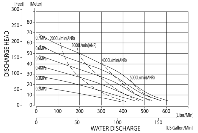
■ NDP-50BAT/BST/BFT
