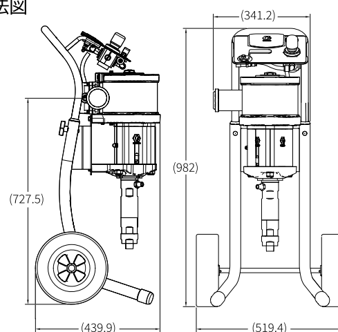
◎ 寸法図
